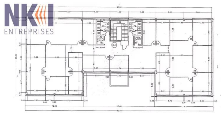
BAT 2 - PLAN NIVEAU 1
